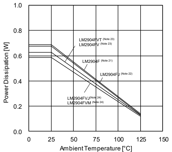
(d) LM2904xxx*2
