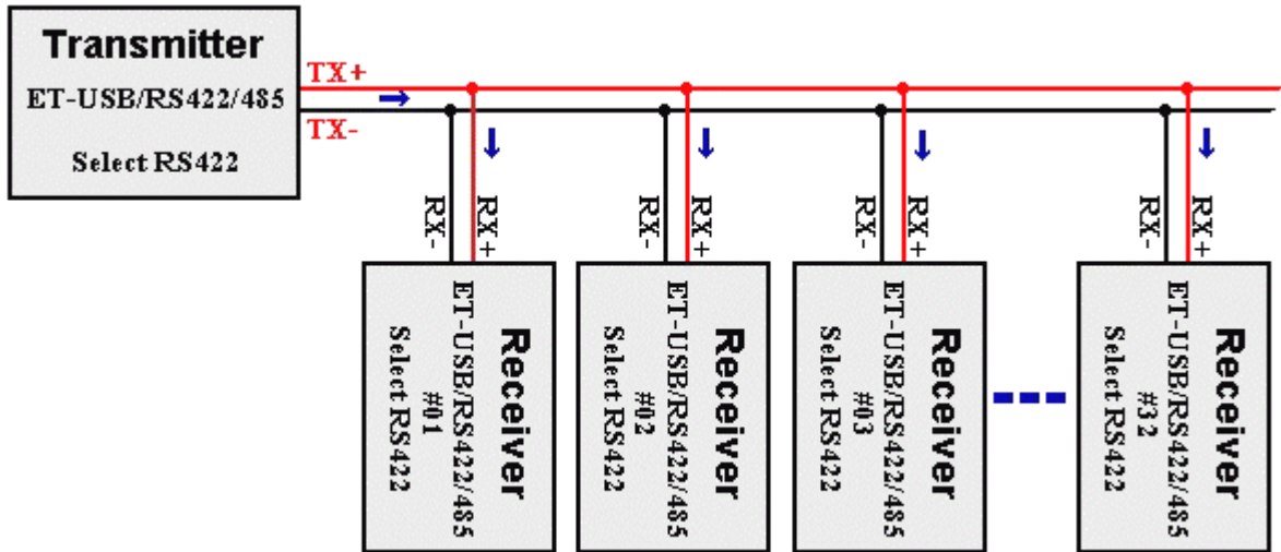
รูปแสดง การต่อสาย RS422 แบบรับหลายตัวพร้อมกัน
