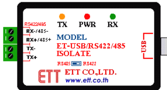
รูปแสดง ET-USB/RS422/485 ISOLATE Module
