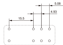
DRPB-1CH/2C
