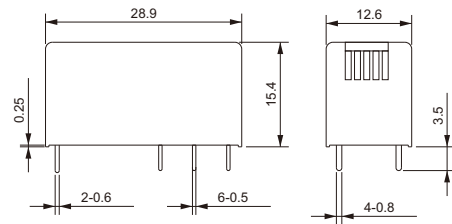
DRPB-1CH/2C
