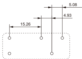
DRPB-1C
