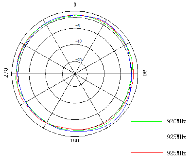
垂直面方向图 Vertical Pattern
