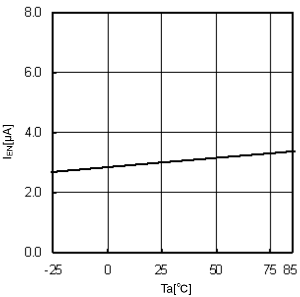
Fig.12 T_a - I_{EN}
