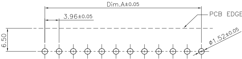
P.C.B Layout
