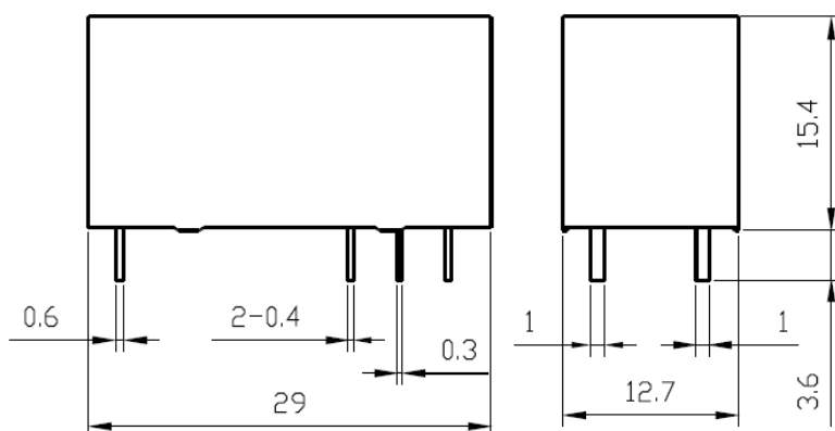
安装孔位图 (底视图)
