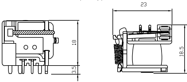
敞开型 Open type
