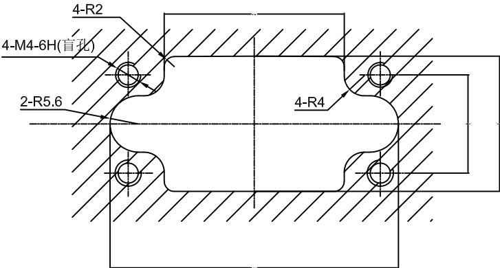
推荐面板开孔尺寸
