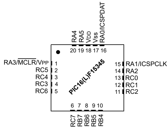
20-PIN UQFN/VQFN/QFN (4x4)
