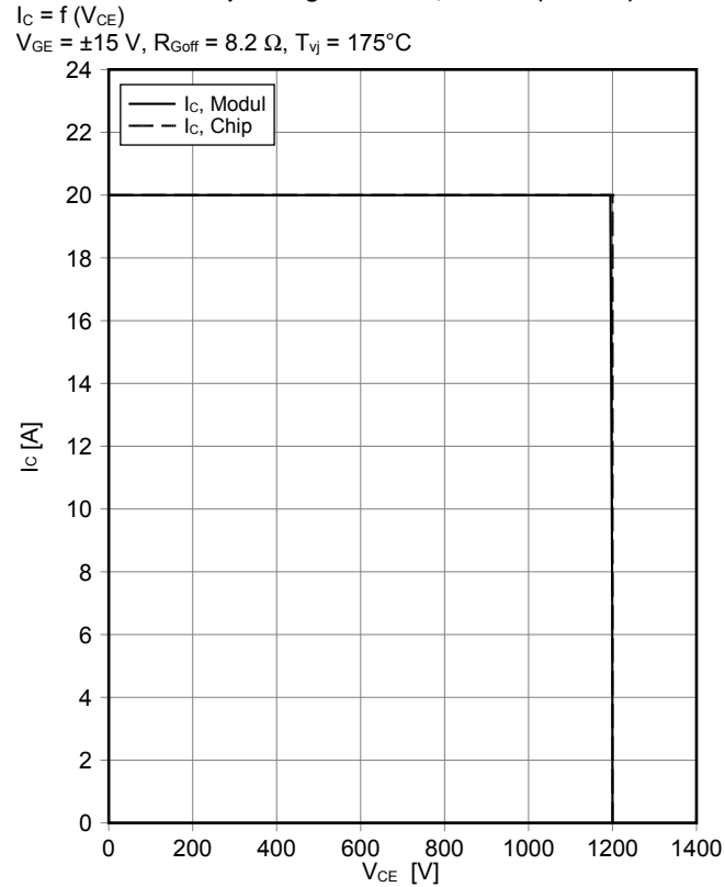
Sicherer Rückwärts-Arbeitsbereich IGBT, Wechselrichter (RBSOA) reverse bias safe operating area IGBT, Inverter (RBSOA)
