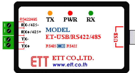
รูปแสดง ET-USB/RS422/485 Module
