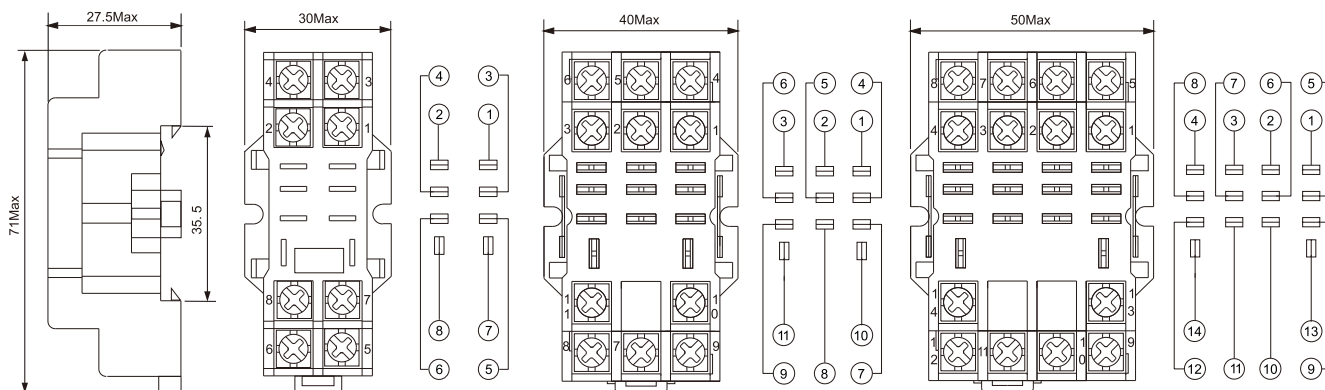
DPTF08A2-3
