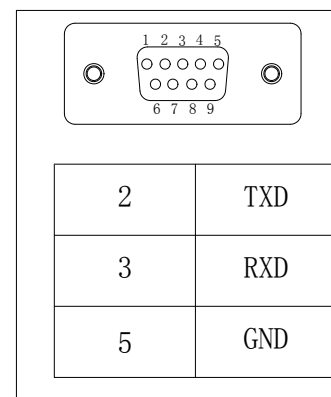
PC DB9 PIN
