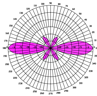
垂直方向图
