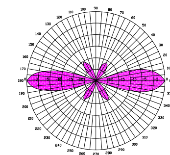
垂直方向图
