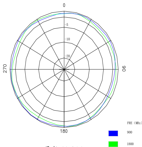
垂直面方向图 Vertical Pattern
