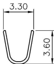
A-A SEC
