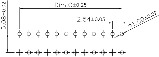
P.C.B Layout
