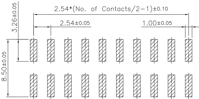
P.C.B Layout
