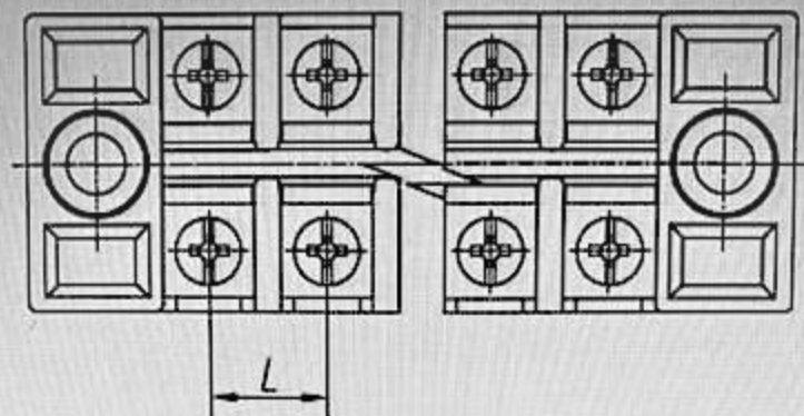
TB系列接线端子相邻极尺寸
