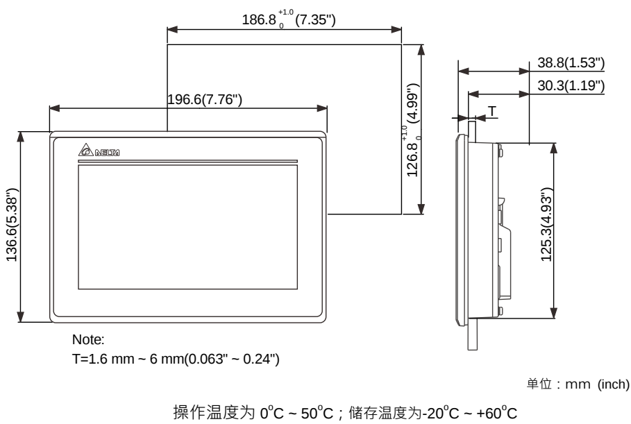
DOP-107PV
