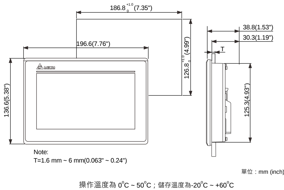
DOP-107PV
