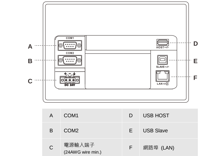
DOP-107PV (背面)
