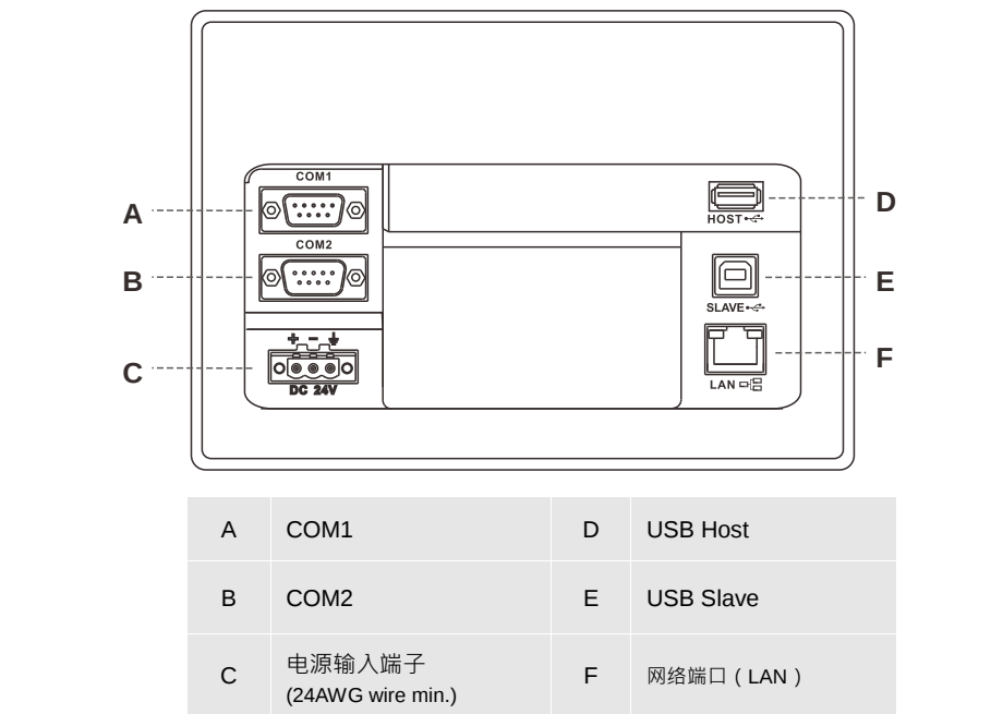
DOP-107PV (背面)
